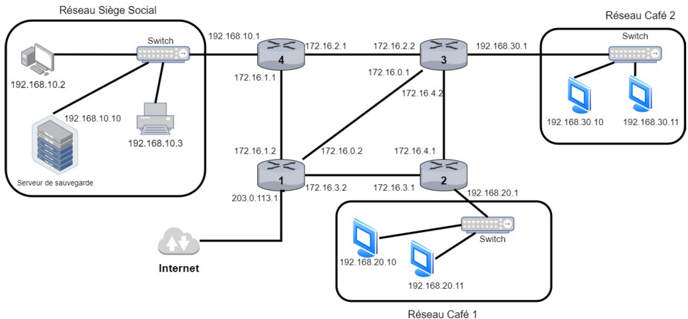
FIGURE 1 – Schéma d'une partie du réseau
