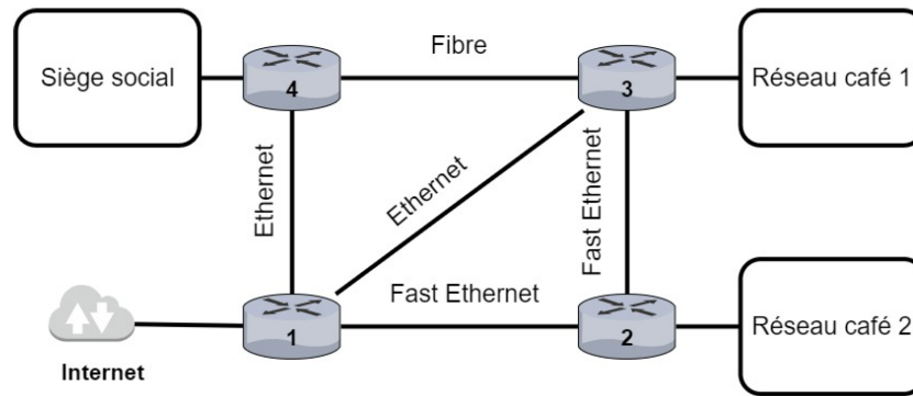
FIGURE 2 – Schéma des types de connexion
